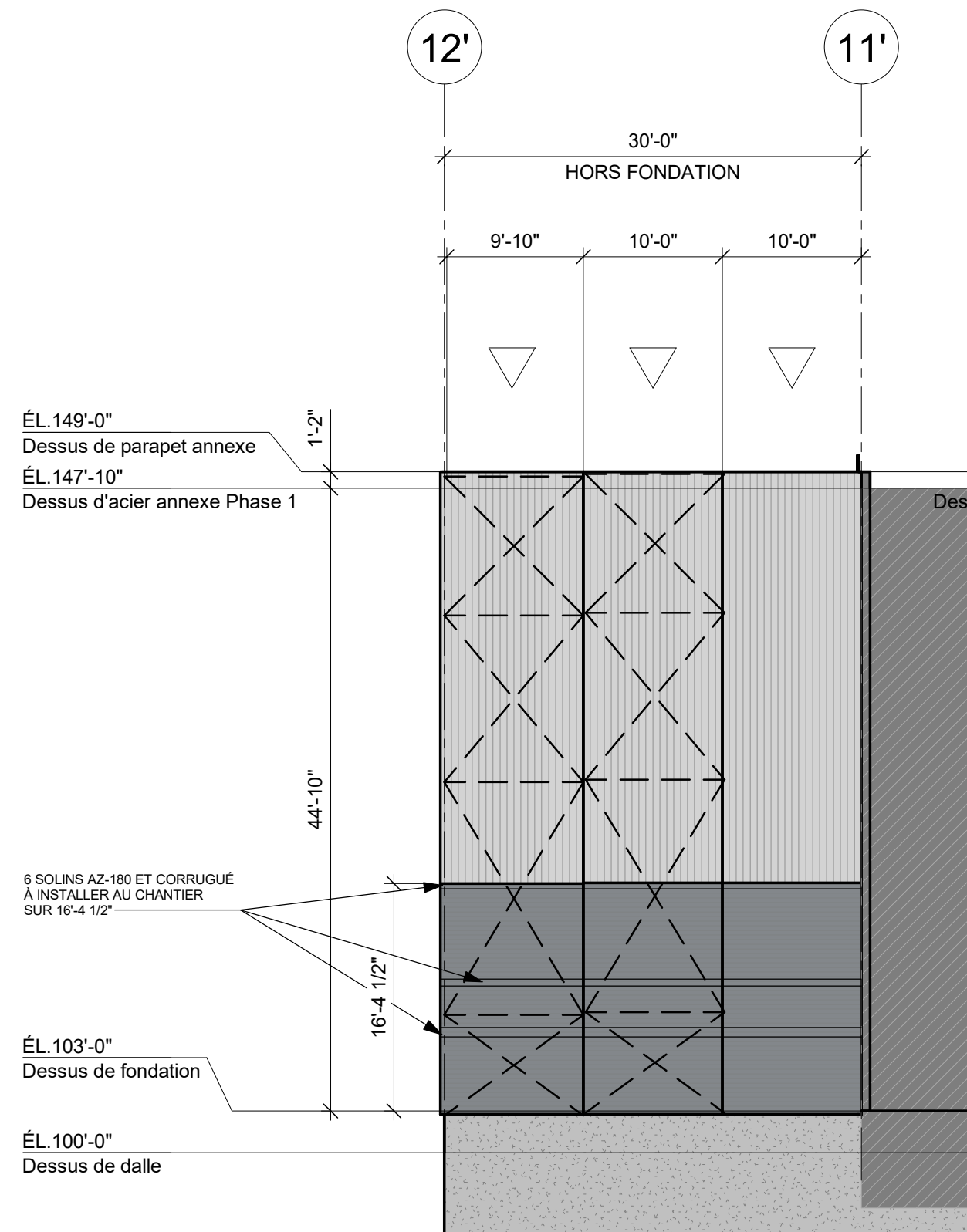
ÉLEVATION AXE D (SUD) 3/32" = 1'-0"
