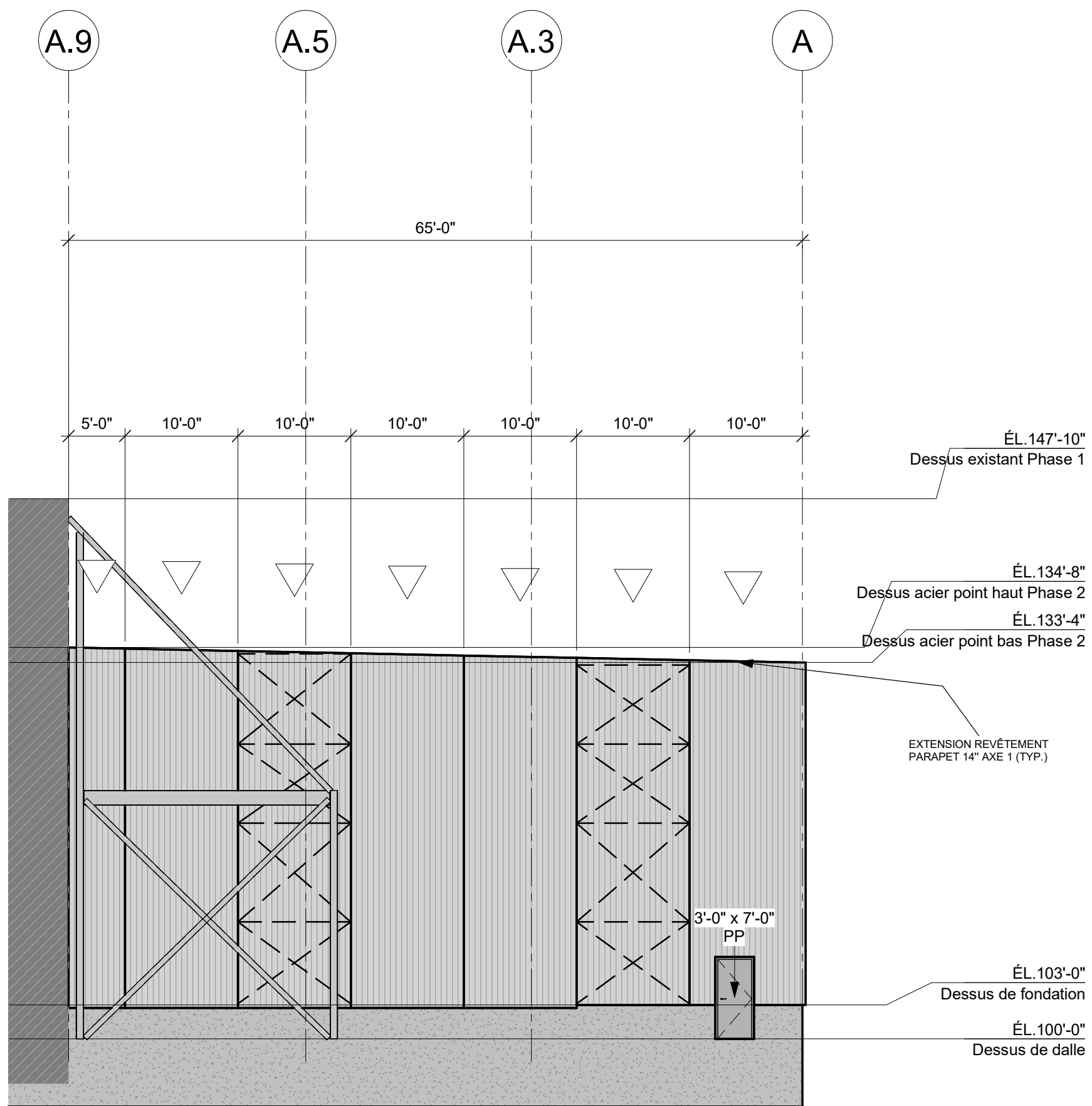
ÉLEVATION AXE 1 (EST) 3/32" = 1'-0"
